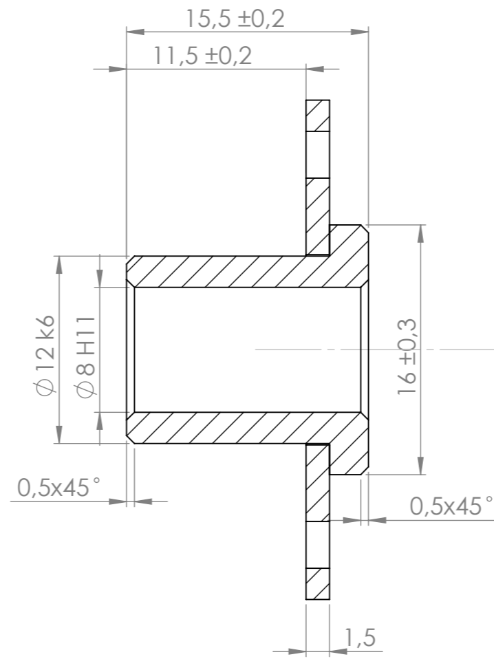
ŘEZ A-A
